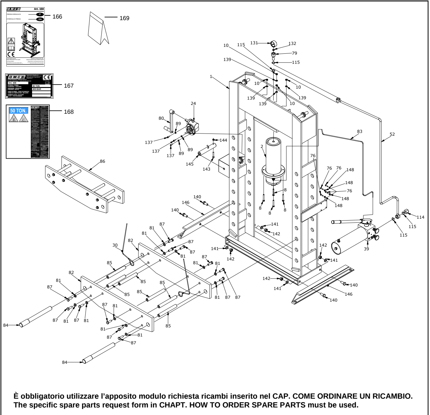
COMPLESSIVO PRESSA PRESS UNIT
